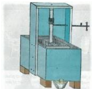
Fig. 55b. Slyng med snoretræk. Træk i håndtaget s, akslen snurrer rundt, og vikler selv snoren op om sig. Så trækker man igen og bliver ved, indtil honningen er slynget ud. Under slyngen ses en honningspand. (Bojesen 1873).
